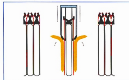
全自动刮刀装置
