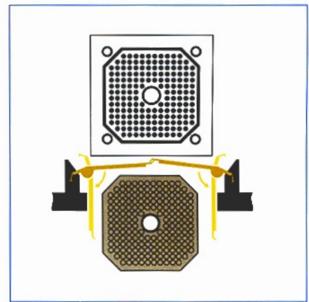
自动集水盘
