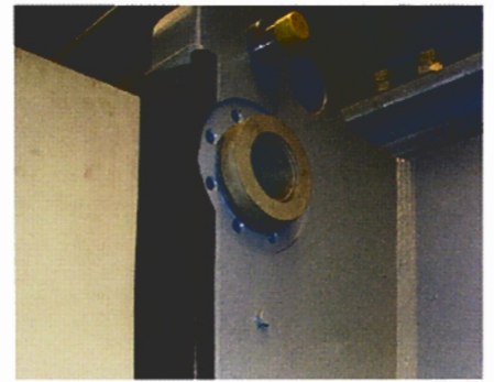
所有湿润表面橡胶包覆 用于强腐蚀应用领域，例如稀酸循环
